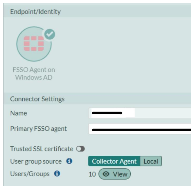
Imagen [20]. Configuración Agente FSSO, conectado y dirigido a un servidor puntual.
