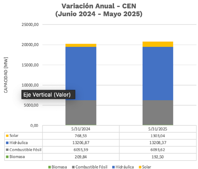
Gráfica 3- Comportamiento de la capacidad efectiva en el último año.
