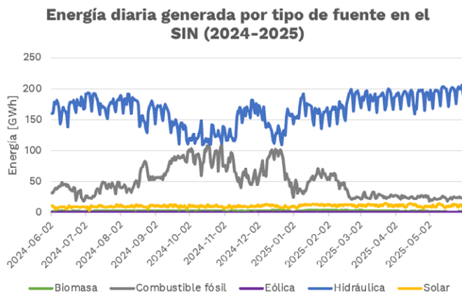
Gráfica 4- Energía generada por tecnología en el último año.
