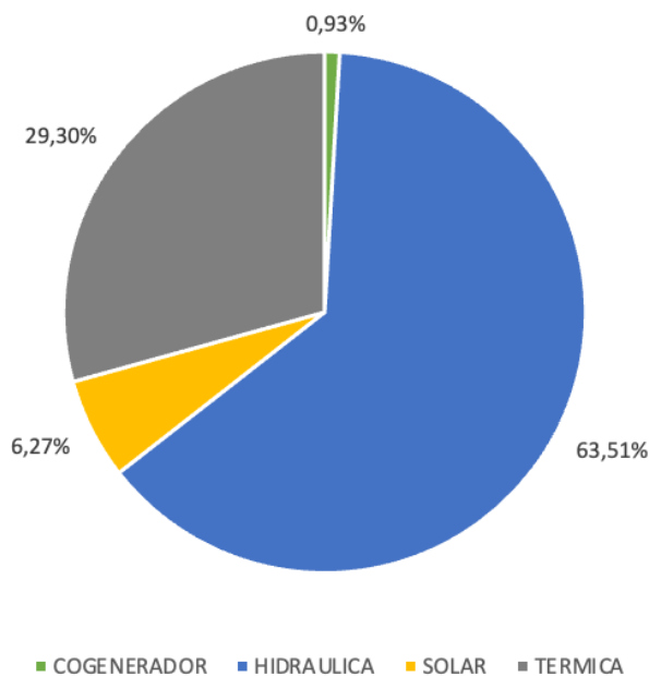
Gráfica 2- CEN a 31 de Mayo de 2025 Capacidad Efectiva Neta - CEN 2025
