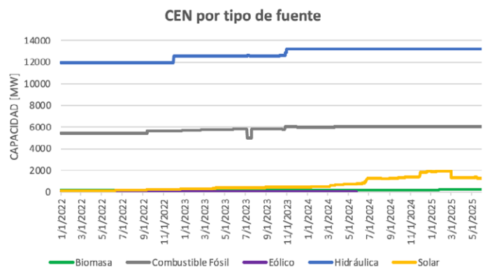
Gráfica 1- CEN por tipo de fuente en el último año
