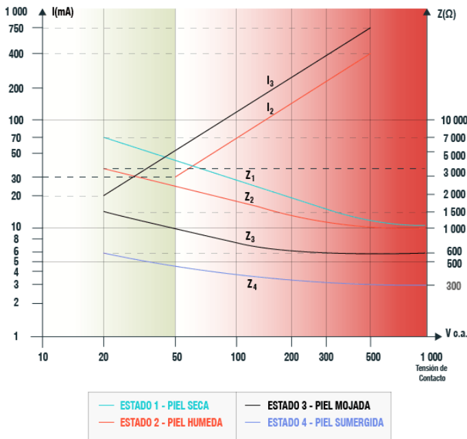
Figura 1.5.1.2. b. Impedancia del cuerpo.
