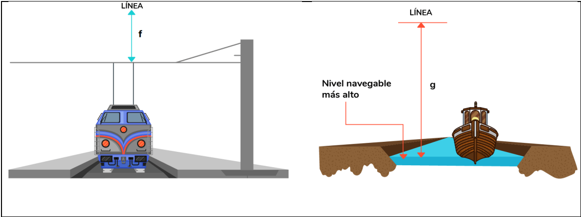
Figura 3.10.2. c. Distancia “f” y “g” para cruces con ferrocarriles y ríos. Fuente: Adaptada de la Resolución 90708 del 2013.
